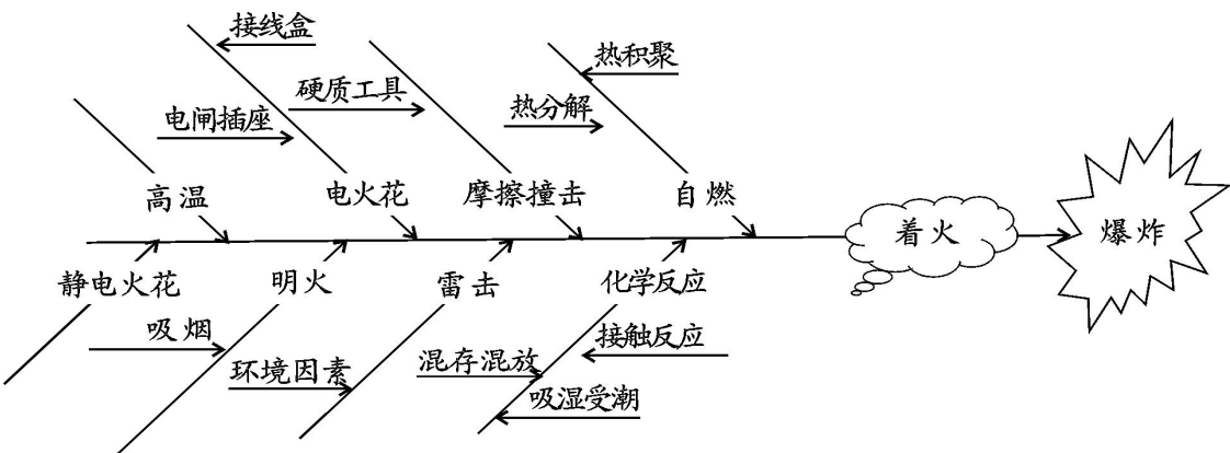
图 3-1 烟花爆竹引爆的因果分析图
